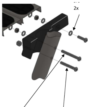
Детайл на закрепването на страничната секция
